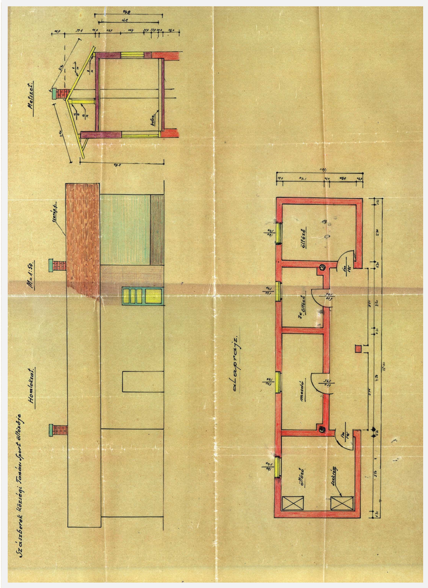
Építési terv, alaprajz
